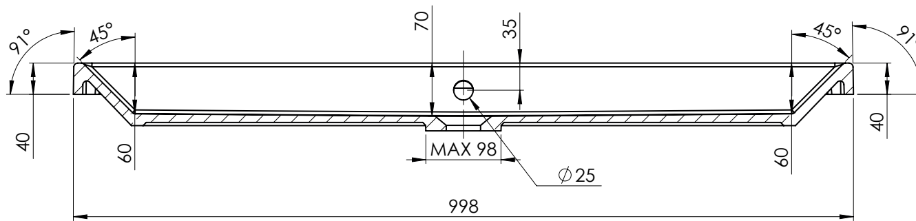
A-A (1 : 5)
