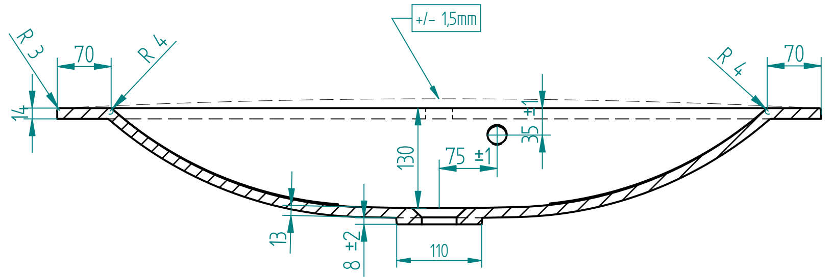
SECTION A-A
