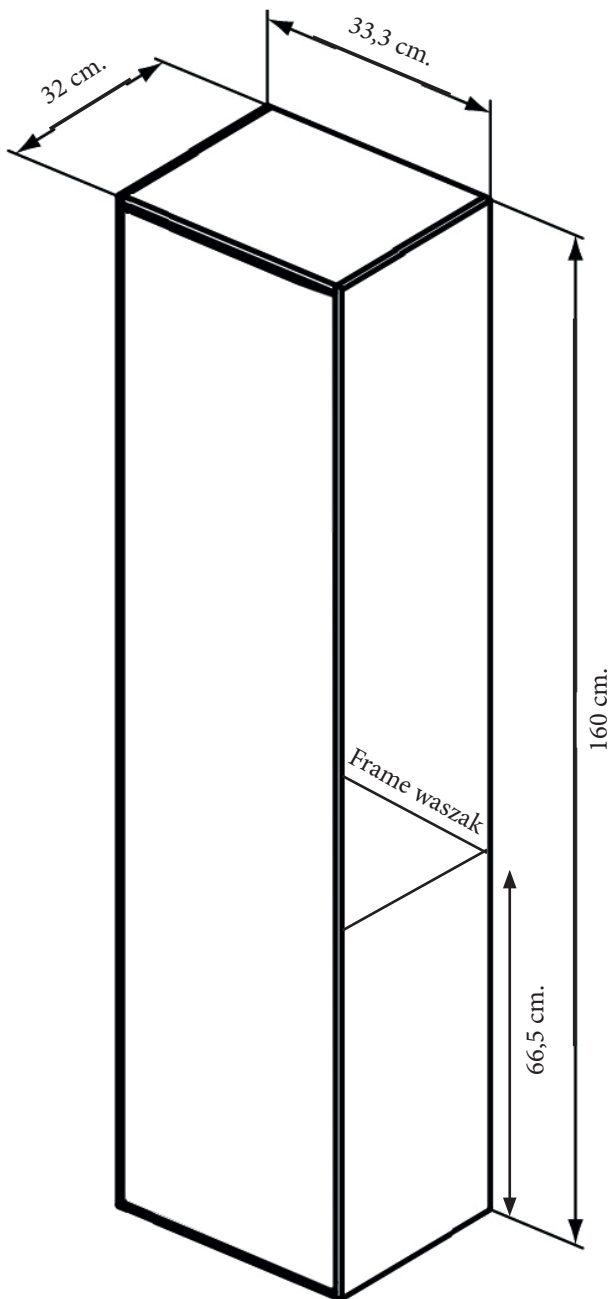
Hoge kolomkast met wasgoedzak (2 planken)
