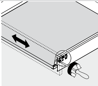
Zijdelingse verstelling
