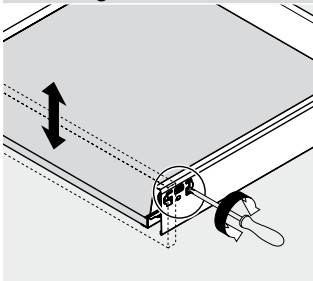
Hoogteverstelling
