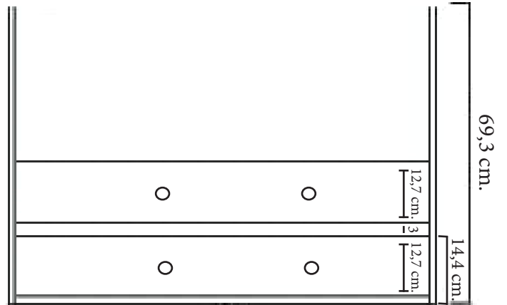
Achterzijde
